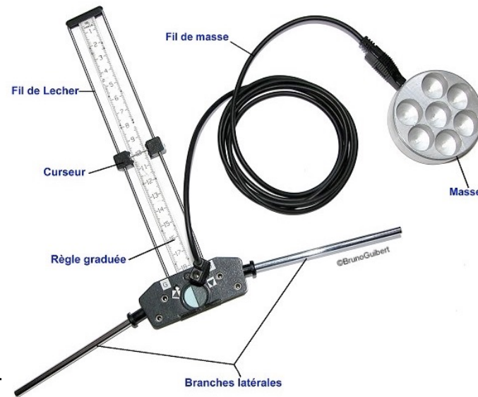
Antenne de Lécher
